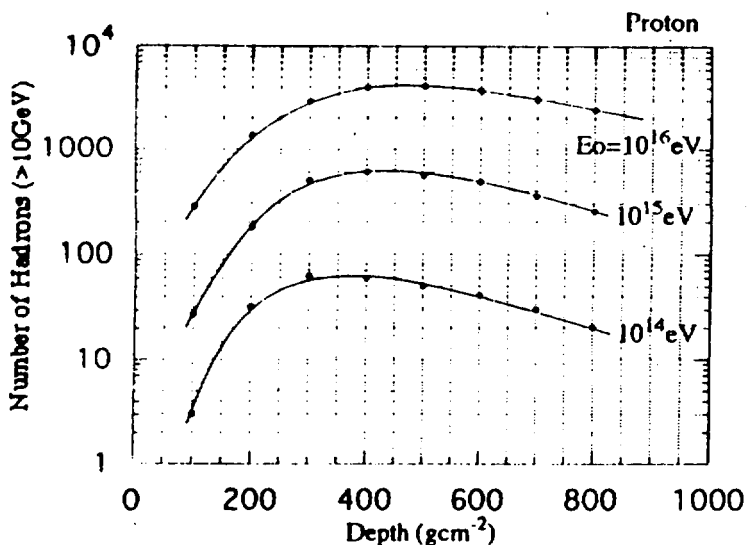
Рис. 5. Изменение числа адронов с E > 10 ГэВ в ливнях, вызванных первичными потоками с энергиями 10^{14} , 10^{15} , 10^{16} эВ при прохождении слоя атмосферы, выраженного в \text{г} \cdot \text{см}^2
