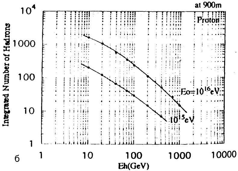
Рис. 6. Энергетический спектр адронов на высоте 5000 м (а), на высоте 900 м (б)
