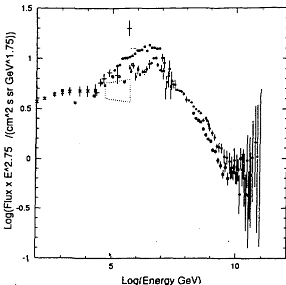
Рис. 3. Дифференциальный энергетический спектр космических лучей [22]
