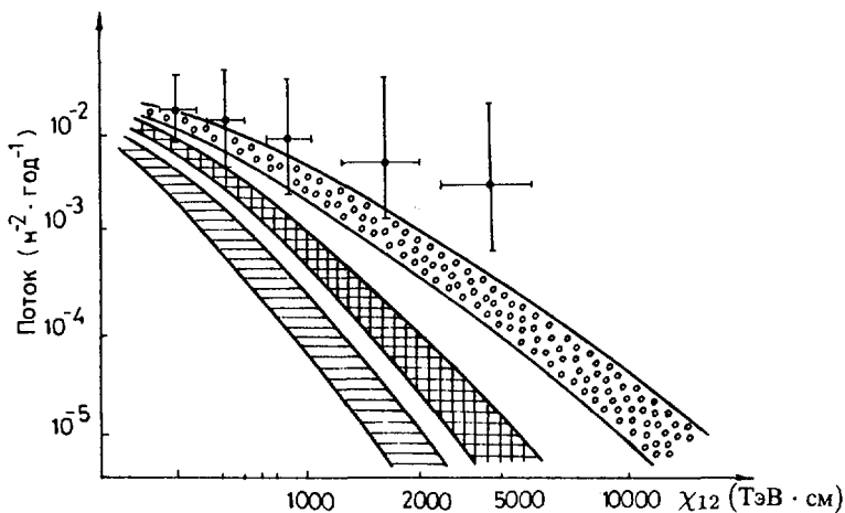
Рис. 9. Интегральный спектр для пяти случаев \gamma -семейств с двойным стволом
